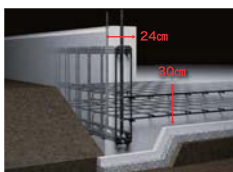
ベタ基礎イメージ
